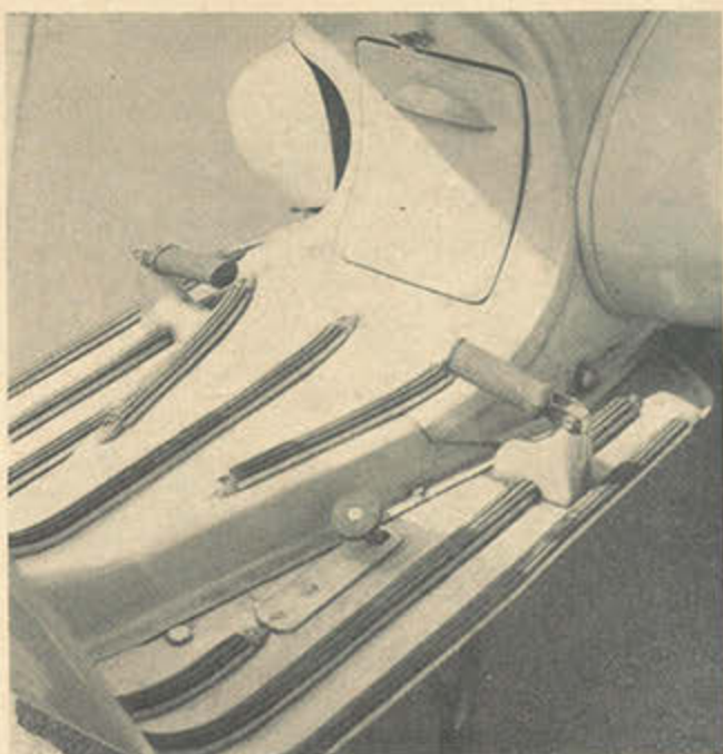
Hier wird die Motorbremse durch einen kleinen Fußhebel ein- und ausgeschaltet. Genau so gut ist es aber möglich, die Motorbremse durch einen kleinen Hebel am Lenker zu betätigen
