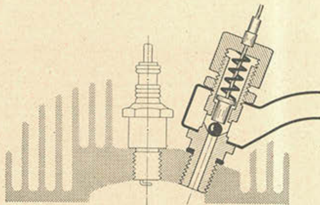
Querschnitt durch eine Vaku-Motorbremse
