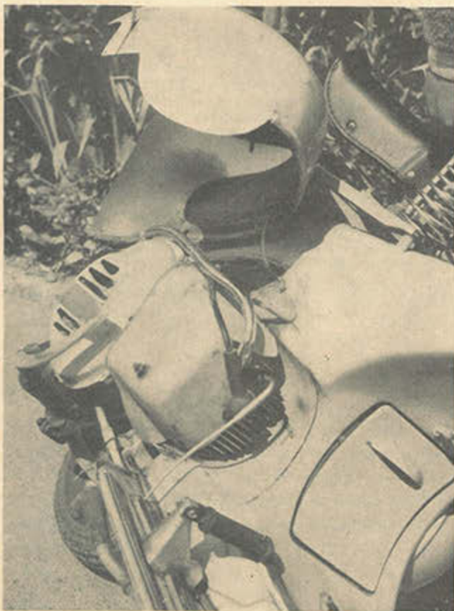
So sieht die fertigmontierte Vaku-Motorbremse an einer Vespa aus. Nach unten läuft der Bowdenzug zum Betätigungshebel. Über den Motor hinweg ist ein kleines Schalldämpferrohr gezogen
