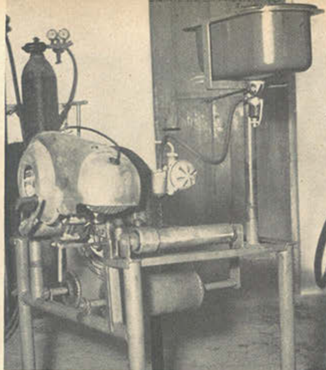
Auf solchen kleinen Prüfständen werden im Messerschmitt-Kundendienst die zu prüfenden Motoren komplett mit dem Hinterrad montiert. Das Hinterrad läuft auf Rollen, der Motor kann also in jedem einzelnen Gang kontrolliert werden.
