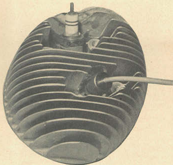
Ein Vespa-Zylinderkopf mit eingebauter Vaku-Motorbremse
